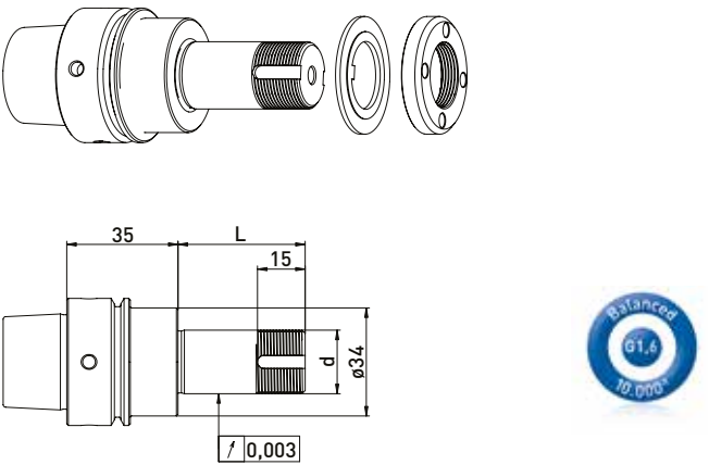
HSK-E40 // \varnothing 20 毫米 // without RS
