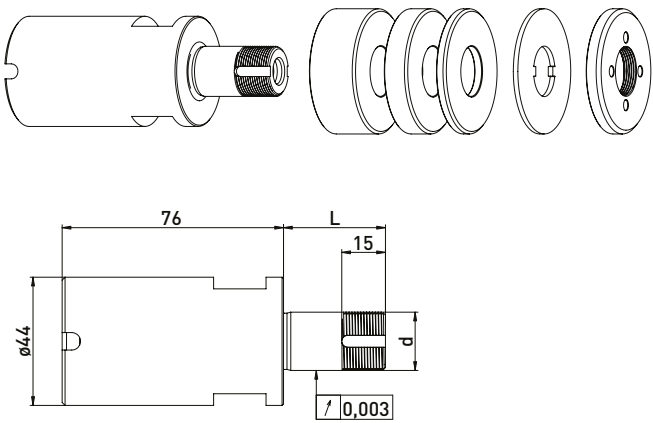
Strausak 内锥 // \varnothing 20 毫米 // RS \varnothing 50 毫米
