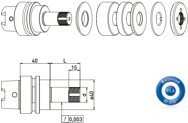
HSK50 // \varnothing 20 毫米 // RS \varnothing 50 毫米
