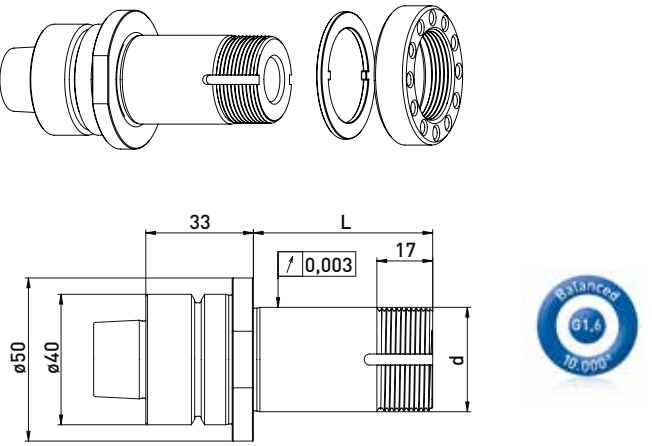
自动 HSK-F40 // \varnothing 32 毫米 // without RS
