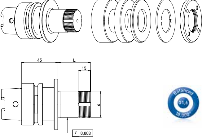
HSK50 // \varnothing 31,75 毫米 // RS \varnothing 60 毫米
