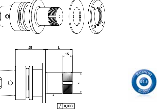
HSK50 // \varnothing 31,75 毫米 // without RS
