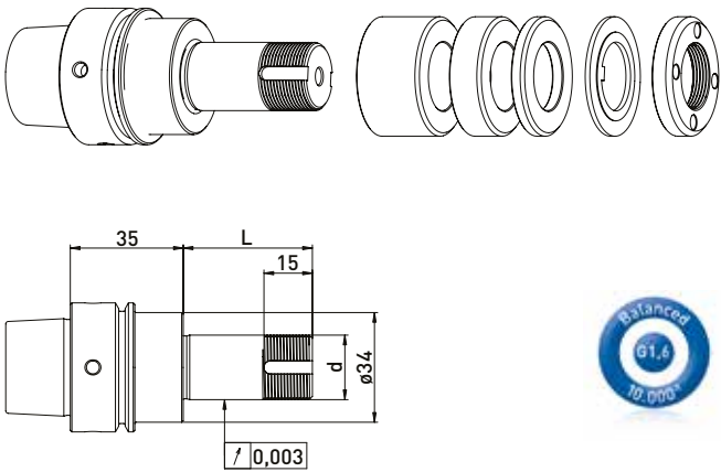
HSK-E40 // \varnothing 20 毫米 // RS \varnothing 35 毫米
