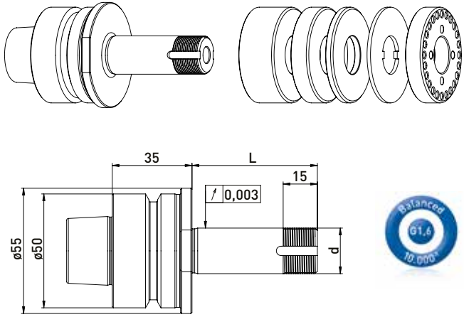
自动 HSK-F50 // \varnothing 20 毫米 // RS \varnothing 50 毫米
