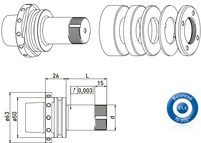
HSK-E50 // \varnothing 31,75 毫米 // RS \varnothing 60 毫米
