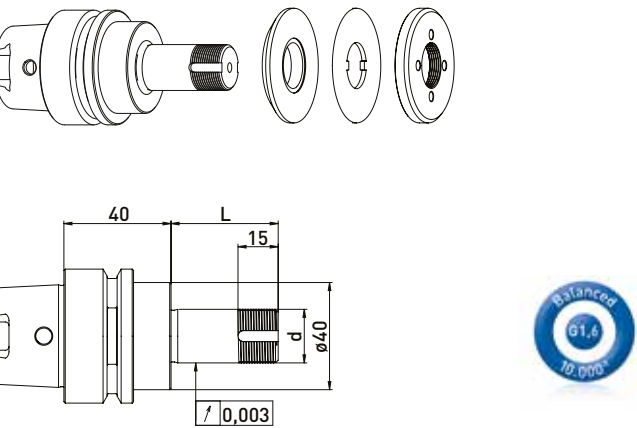
HSK50 // \varnothing 20 毫米 // without RS
