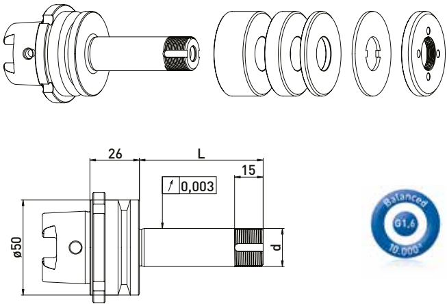
HSK50 // \varnothing 20 毫米 // RS \varnothing 50 毫米
