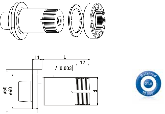
手动 HSK-F40 // \varnothing 32 毫米 // without RS
