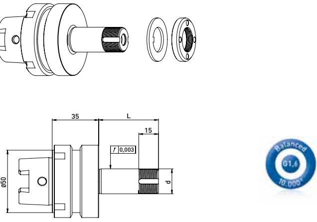
HSK50 NGC // \varnothing 20 毫米 // without RS
