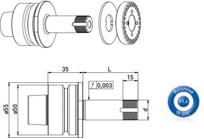
自动 HSK-F50 // \varnothing 20 毫米 // without RS
