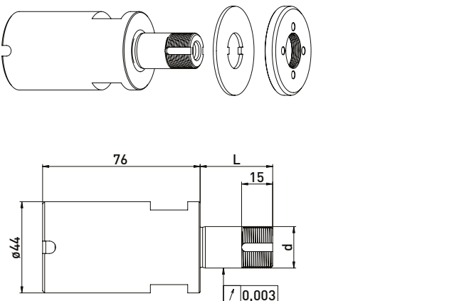
Strausak 内锥 // \varnothing 20 毫米 // without RS
