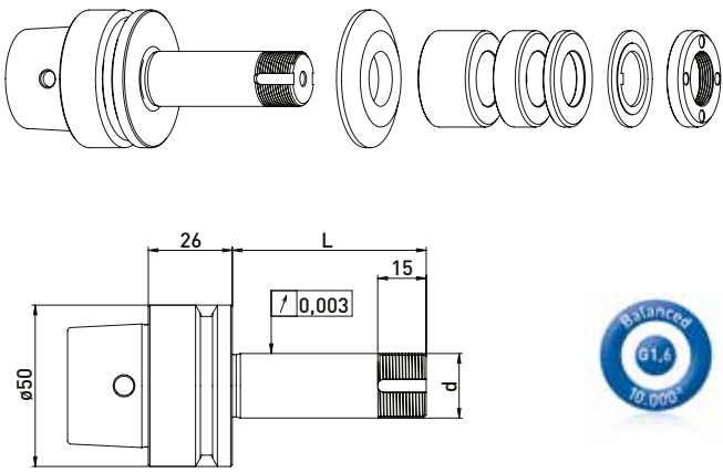
HSK-E50 // \varnothing 20 毫米 // RS \varnothing 35 毫米
