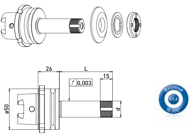
HSK50 // \varnothing 20 毫米 // without RS
