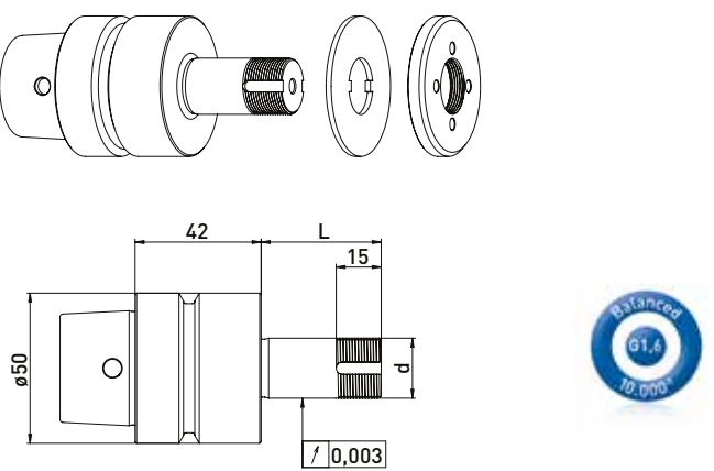
HSK-E50 // \varnothing 20 毫米 // without RS
