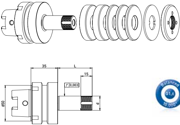
HSK50 NGC // \varnothing 20 毫米 // RS \varnothing 50 毫米
