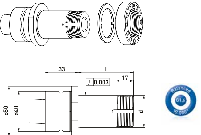
自动 HSK-F40 // \varnothing 31,75 毫米 // without RS
