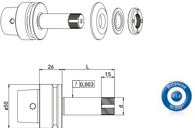
HSK-E50 // \varnothing 20 毫米 // without RS
