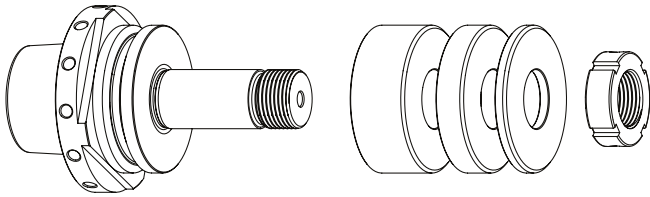
GWA HSK-E50 // ø20 mm // RS ø50 mm
