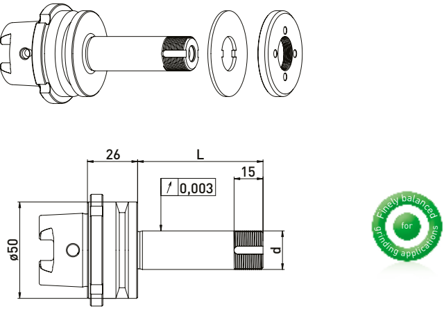
GWA HSK50 // ø20 mm // without RS
