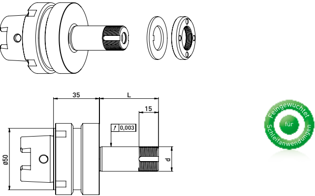
GWA HSK50 NGC // ø20 mm // without RS
