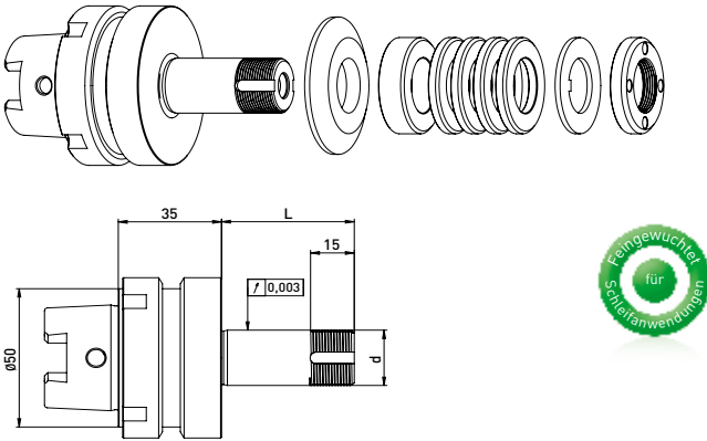
GWA HSK50 NGC // ø20 mm // RS ø35 mm
