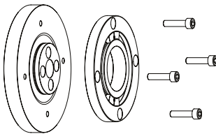
GWA ø125 // ø50 mm
