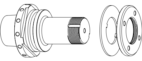
GWA HSK-E50 // ø31,75 mm // without RS
