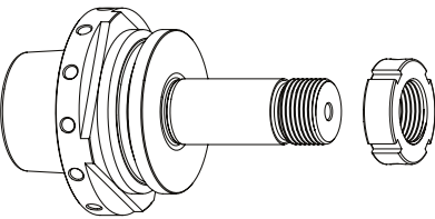
GWA HSK-E50 // ø20 mm // without RS
