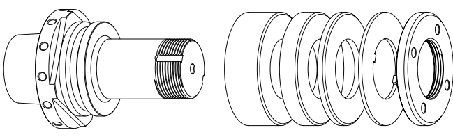
GWA HSK-E50 // ø31,75 mm // RS ø60 mm
