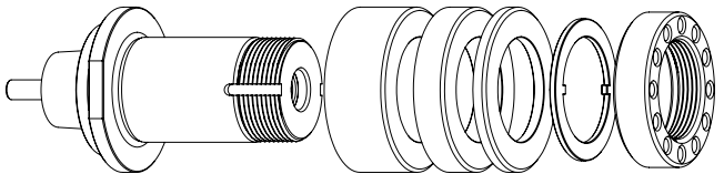
GWA manual HSK-F40 // ø31,75 mm (1¼) // RS ø50 mm
