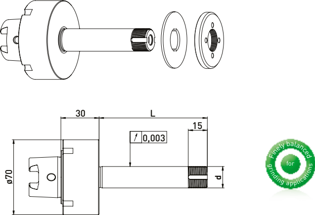
GWA HSK50 // ø20 mm // without RS
