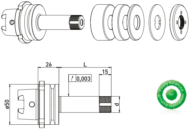
GWA HSK50 // ø20 mm // RS ø50 mm
