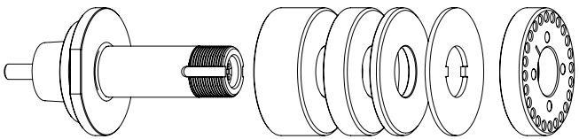
GWA manual HSK-F40 // ø20 mm // RS ø50 mm
