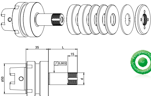
GWA HSK50 NGC // ø20 mm // RS ø50 mm
