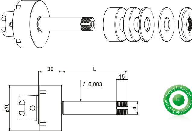
GWA HSK50 // ø20 mm // RS ø50 mm
